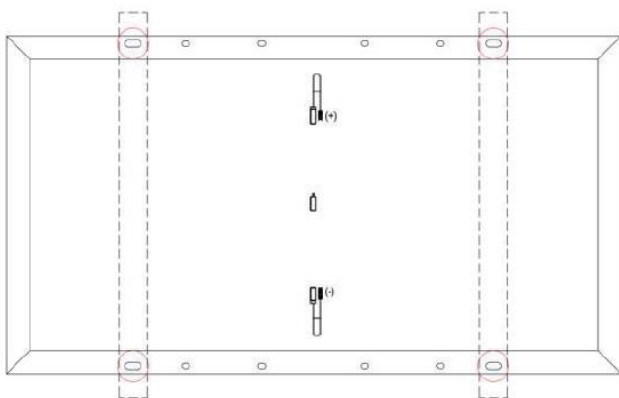
Figure 3 : Installation des modules avec boulons. Rail perpendiculaire au côté long.
