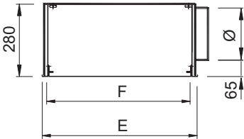
NEXT-KLIN & MID NEXT-KLIN piquage latéral
