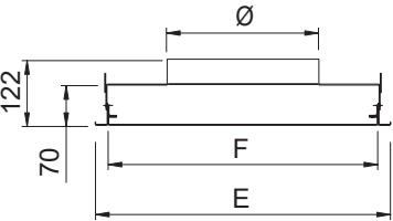
NEXT-KLIN & MID NEXT-KLIN piquage supérieur (Hauteur sous plafond minimum 400 mm)
