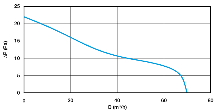
Courbe aéraulique DESIGN 100
