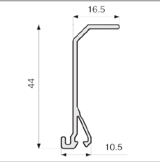
SEP-C 55 - Cloison de séparation Dimensions
