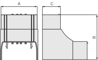
NIAV - Angle intérieur variable Dimensions
