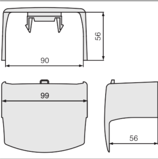
NTAC 90 - Té de dérivation TA-C Dimensions
