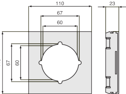
CSA-60 - Boîtier d'appareillage Entraxe 60 Dimensions
