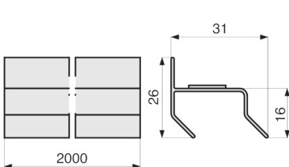
DST - Joint de sol rehausseur Dimensions
