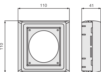
CSA-CE - Boîtier d'appareillage Prise CE Dimensions
