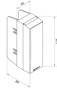
SUPPORTDISJ - Boîtier d'appareillages 2 modules - Dimensions
