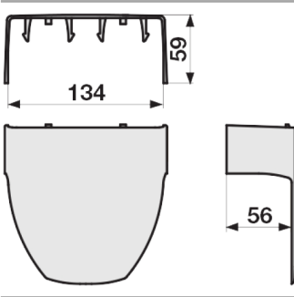
NTAC-134 - Té de dérivation TA-C Dimensions
