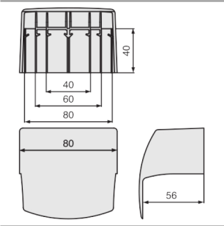
NTAG - Té de dérivation TA-C Dimensions
