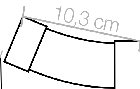
Encombrement coude allongé 22,5°
