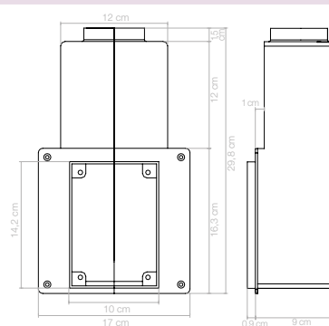
Encombrement contre-prise mur brique pour flexible rétractable
