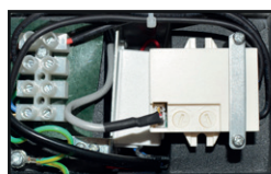
Réglage du détecteur au dos du produit
