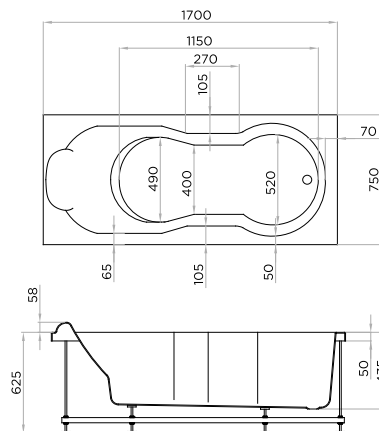
200 litres L 170 x l 75 x P 43,5 x H 62,5 cm
