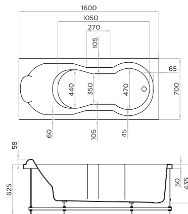
170 litres L 160 x l 70 x P 43,5 x H 62,5 cm
