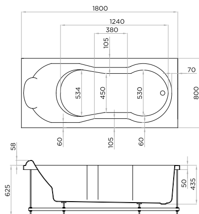
230 litres L 180 x l 80 x P 43,5 x H 62,5 cm
