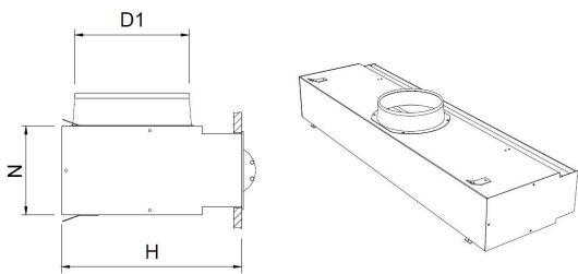
PLKB : Piquage latéral circulaire
