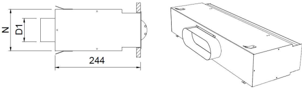
PLKB/S : Piquage supérieur elliptique
