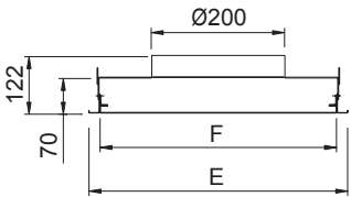
PLAY-KLIN piquage supérieur (Hauteur sous plafond minimum 400 mm)
