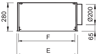
PLAY-KLIN piquage latéral
