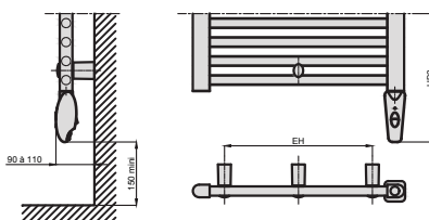
VERSION ELECTRIQUE A LIAISON RF
