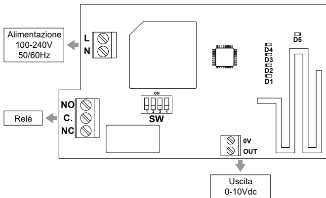
Fig. 1: Scheda elettronica
