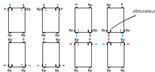
avec obturateur
