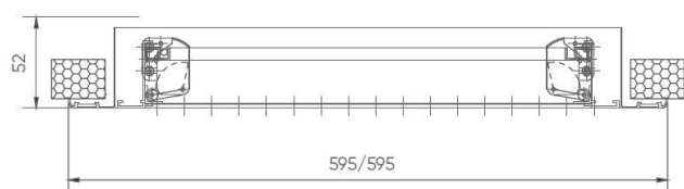
Grille avec filtre sans plénum GRMC-FP/F
