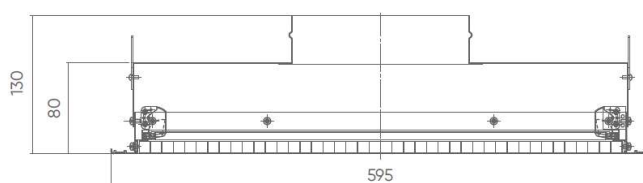
Grille avec plénum monté GRMC-FP/F D 200
