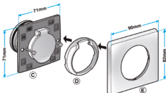
Encombrement prise Celiame
