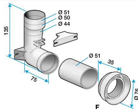
Encombrement contre-prise filaire Celiame
