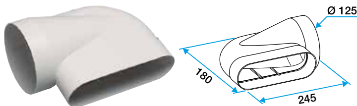
Coude 90° horizontal pour conduit
