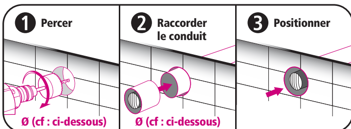
MONTAGE MURAL
