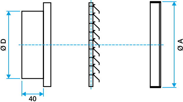
Grille AR 637 diamètre 125 à 315 mm
