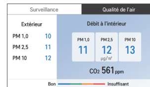
Écran « Qualité de l'air » de la ventilation
