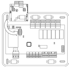
Connexion de la passerelle AZX8GAW / AZX6GAW à l'AZX6CCPGAWI
