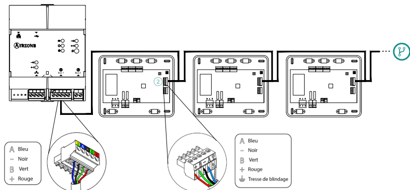
AZX6WSPHUB depuis une unité centrale du système vers d'autres unités centrales
