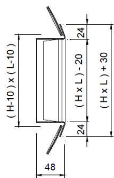
GCF/S : Grille seule simple déflexion
