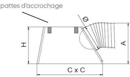
Plénum BOXSTAR
