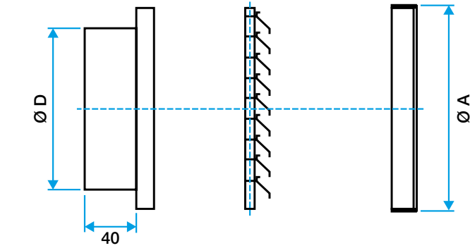
Grille AR 637 diamètre 125 à 315 mm
