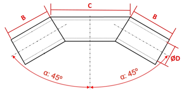
Schéma dimensions
