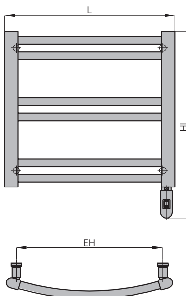
VERSION ÉLECTRIQUE
