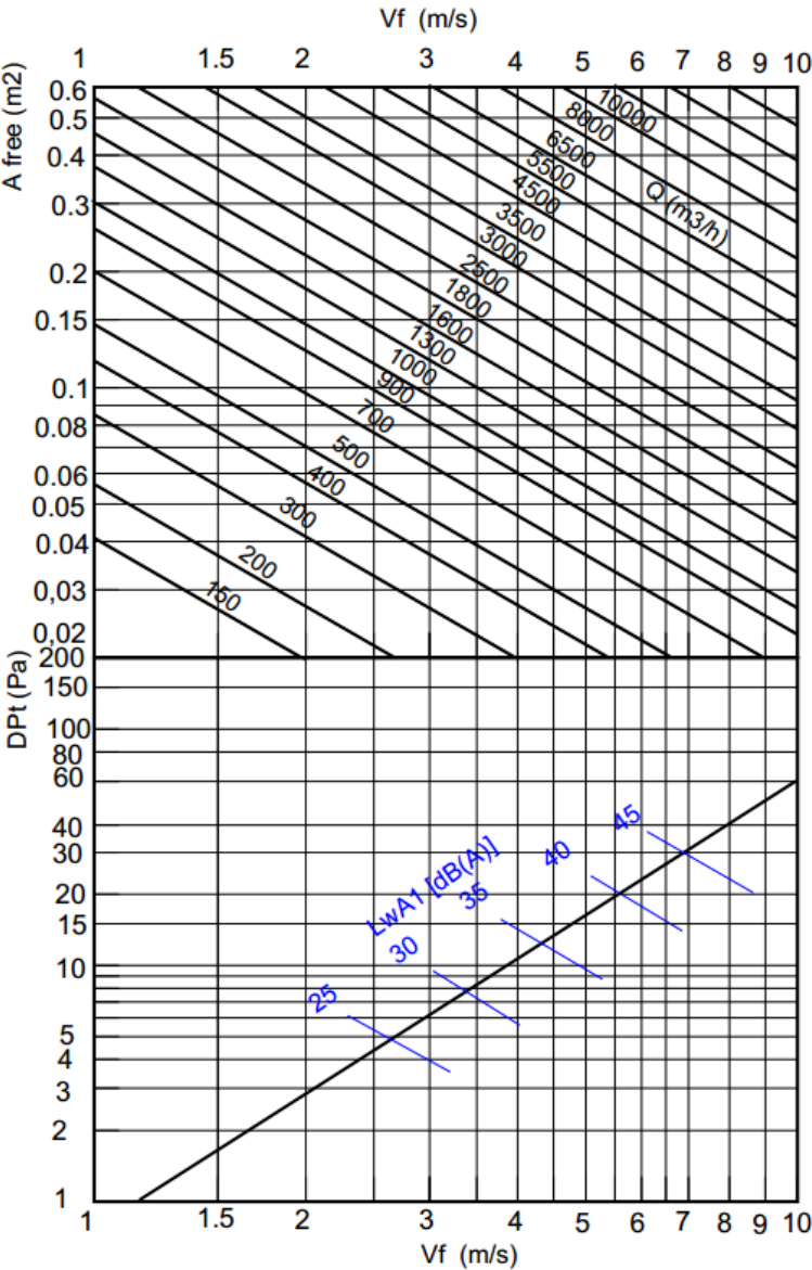
VITESSE LIBRE / PERTE DE CHARGE / PUISSANCE SONORE
