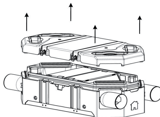
Conduit isolé
