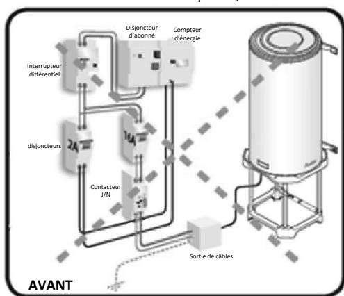
Branchement standard d'un chauffe-eau électrique HC/HP
