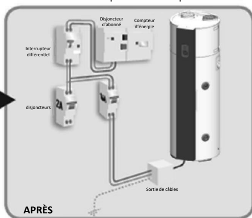
Installation du chauffe-eau branchement permanent uniquement
