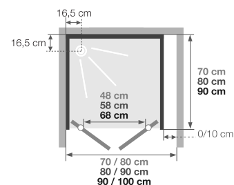
Installations réversibles gauche / droite
