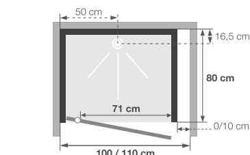
Kineprime Glass C90 niche - version mécanique - 2 portes pivotantes
