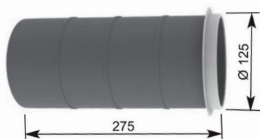
Manchon traversée de dalle :
