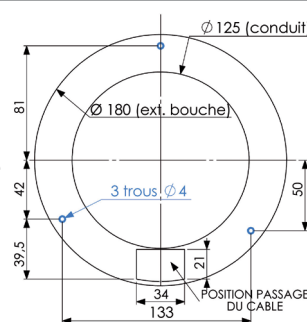
Schéma platine
