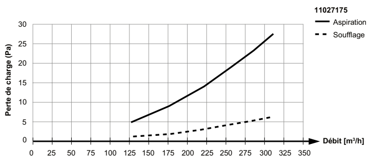
Caisson OPTIFLEX 16 piquages - Courbes de pertes de charge
