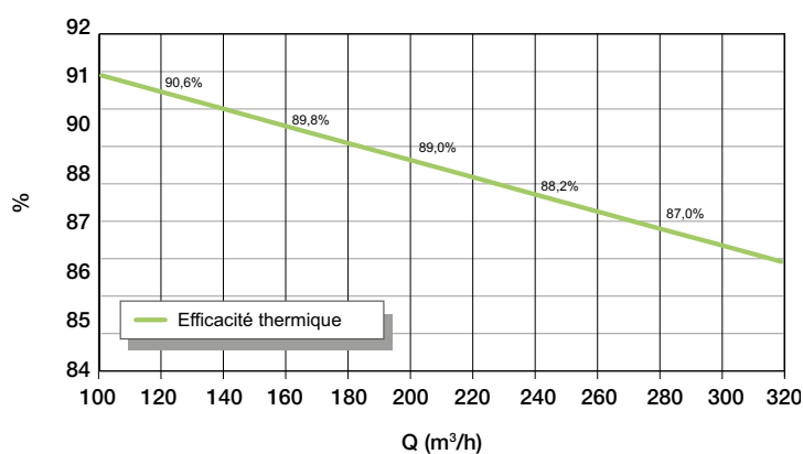
Efficacité thermique InspirAIR® Side 300 Classic
