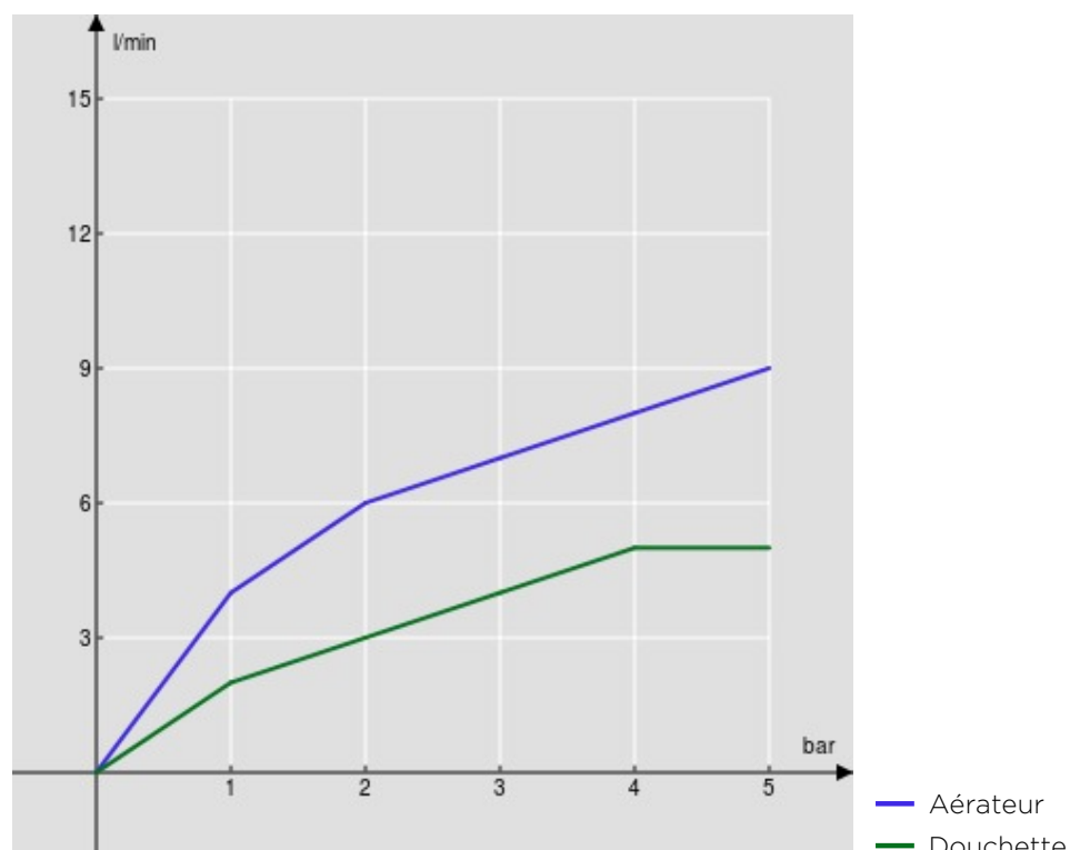
GRAPHIQUE DE DÉBIT: CHAUDE/FROIDE
