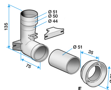
Encombrement contre-prise filaire Celiene
