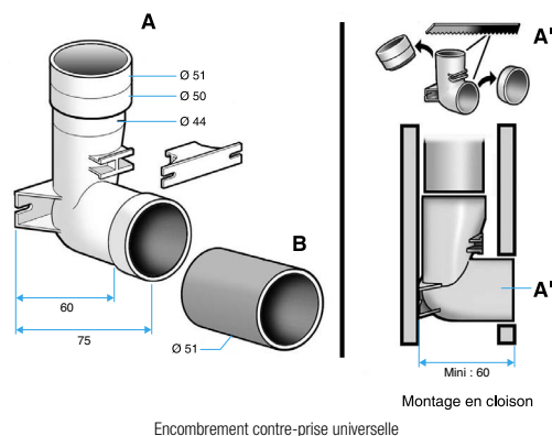
Encombrement contre-prise universelle
