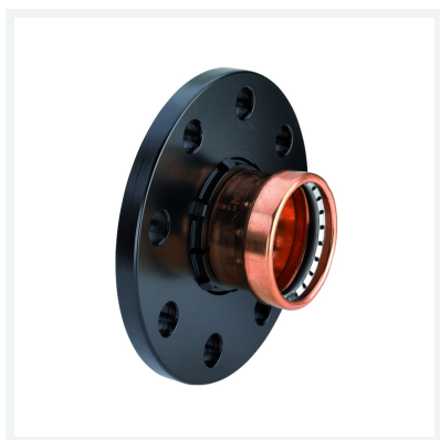
Profipress XL-Raccord à bride avec SC-Contur modèle 2459.5XL article 534 042
