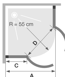
Smart Design R/P sans seuil - profilé chromé
